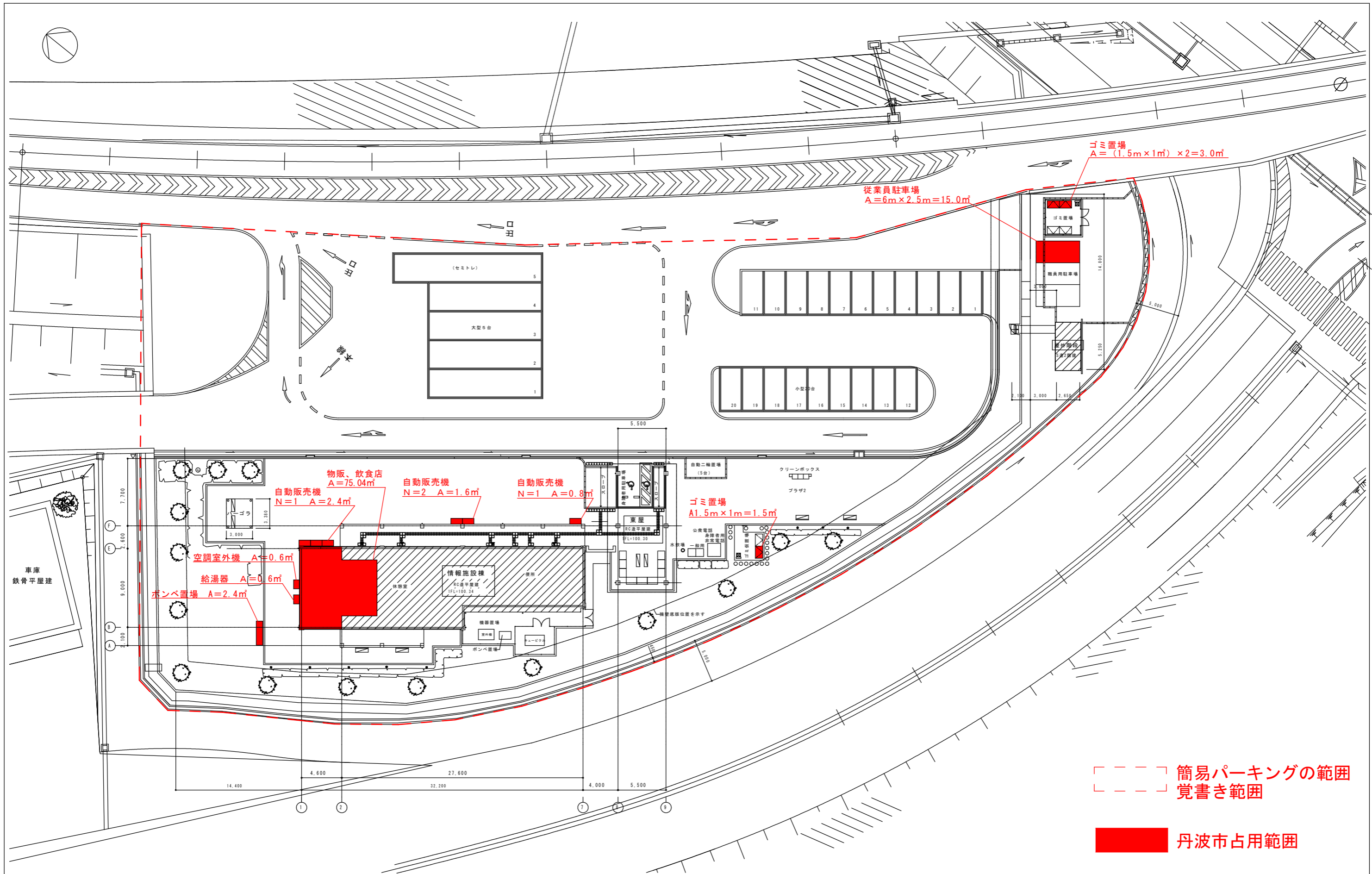
簡易パーキング氷上平面図
