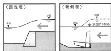
水位の低減効果がある転倒井堰 ※アグレッシブたんば Vol.11 より
