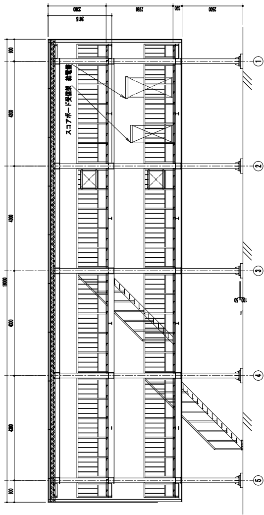
背面図
